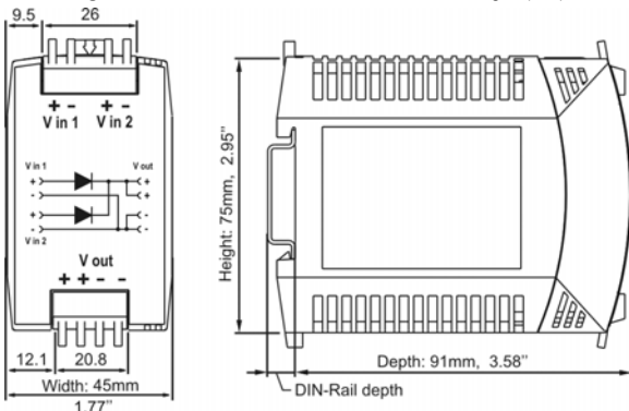
Fig. 7 / Bild 7 MLY02.100: Dimensions / Abmessungen (mm)
